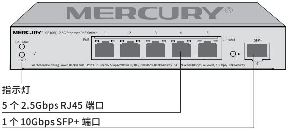
图 2-4 SE106P 前面板示意图
