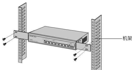
图 3-3 机架安装示意图
