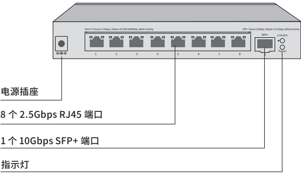
图2-5 SE109后面板示意图
